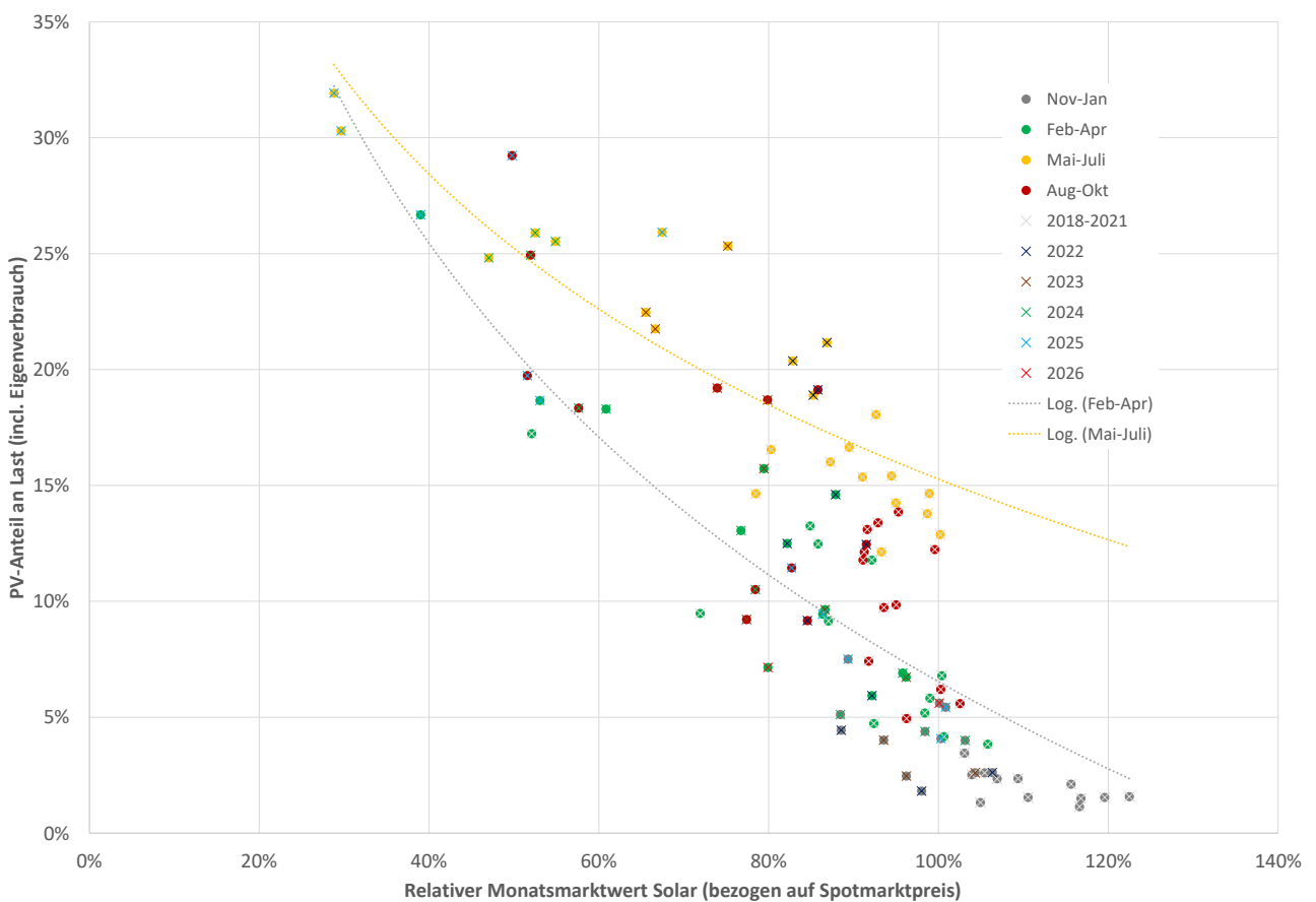
PV-Anteil vs. Marktwert (Monatsbasis)
