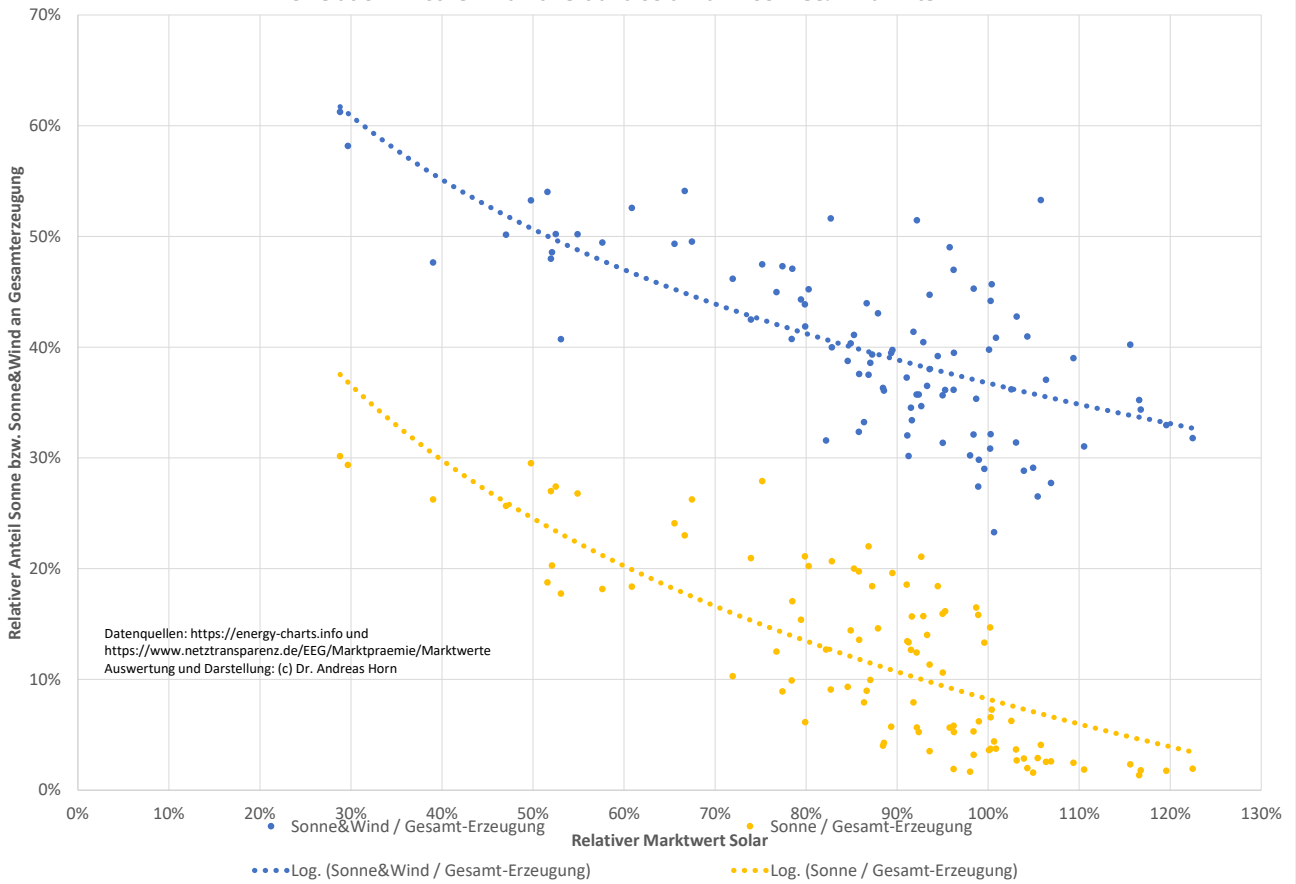
Korrelation zwischen Marktwert und Solar- bzw. Sonne&Wind-Anteil
