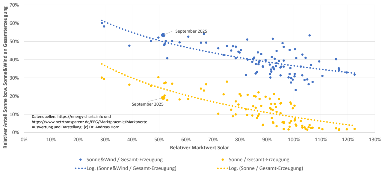
Korrelation zwischen Marktwert und Solar- bzw. Sonne&Wind-Anteil
