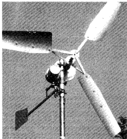
Windag-Windenergiekonverter mit 1,8 m Rotordurchmesser
