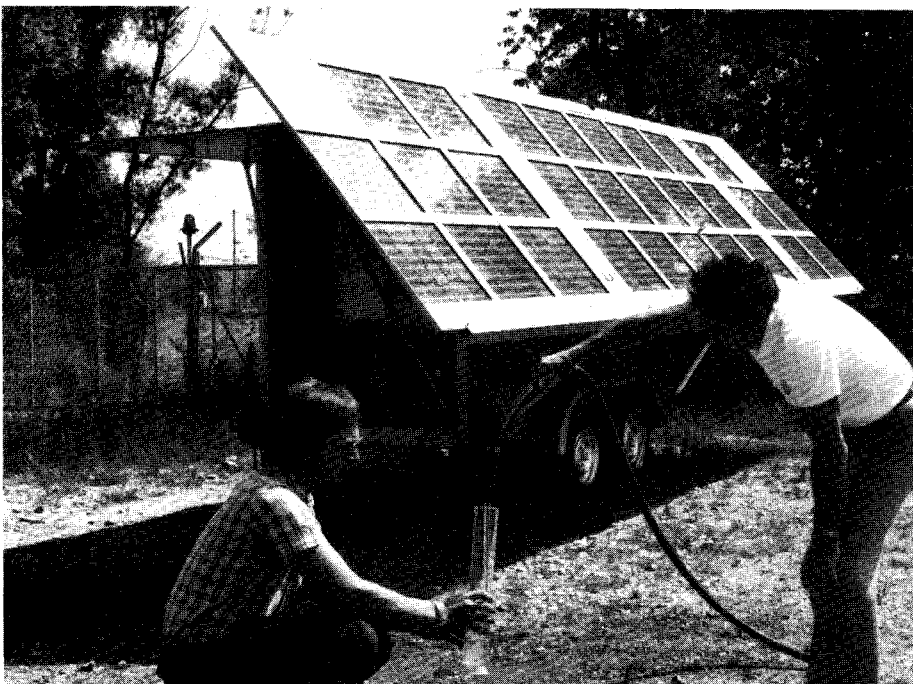
Mobile, mit Solarstrom betriebene Wasseraufbereitungsanlage, wie sie von Dornier gebaut und zu Versuchszwecken nach China und Somalia geliefert wurde. Das Solarzellenfeld läßt sich derart zusammenlegen, daß es gemeinsam mit anderen Klappen einen geschlossenen, containerartigen Aufbau bildet, mit dem man über Land fahren kann.
